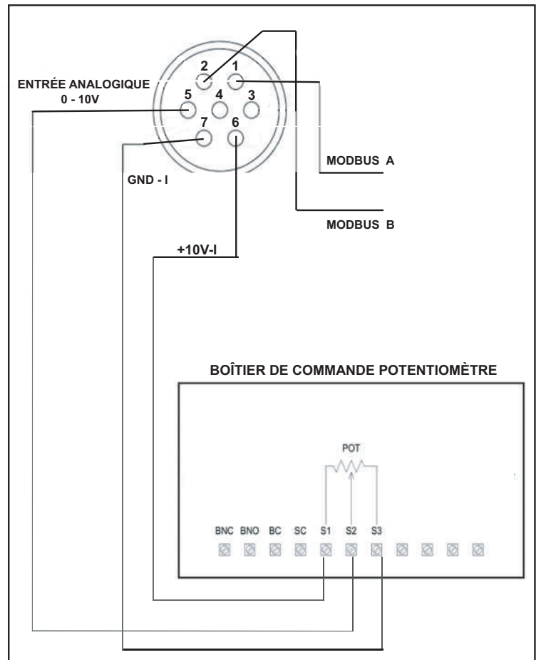
DÉTAIL CONNEXIONS
