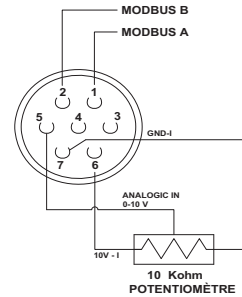
DÉTAIL CONNEXIONS
